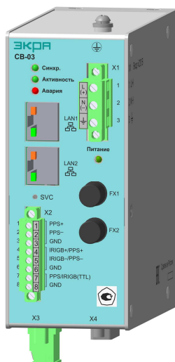
Рисунок 5 – Внешний вид устройства СВ-03 (без исп.)
