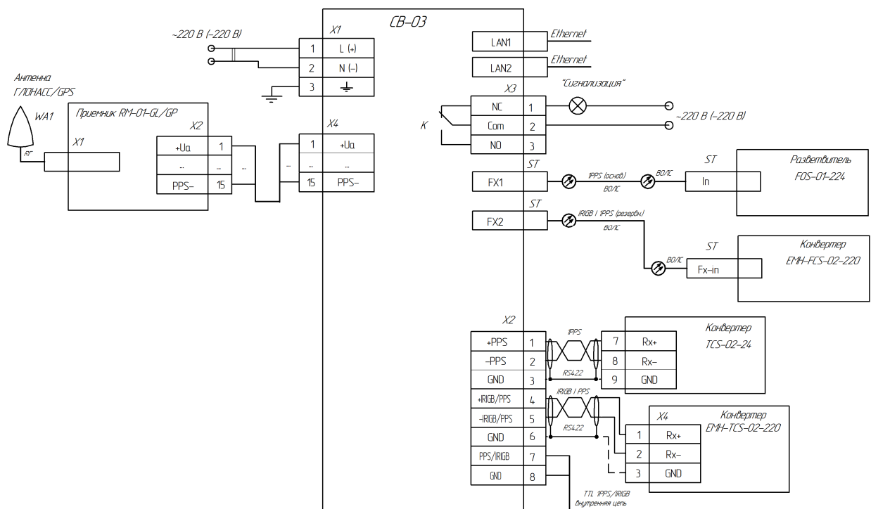
Рисунок 7 – Схема включения устройства СВ-03 (без исп.)
