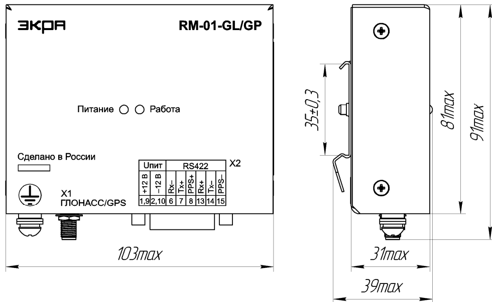
Рисунок 2 – Общий вид приемника RM-01-GL/GP
