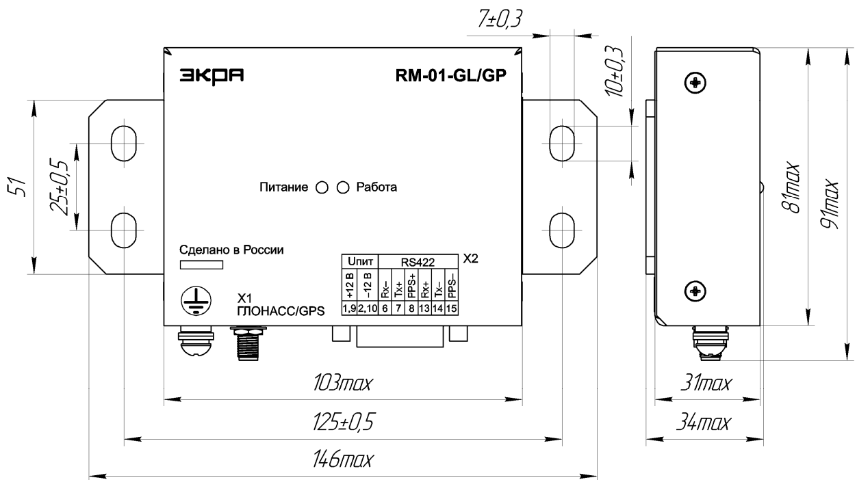
Рисунок 3 – Общий вид приемника RM-01-GL/GP-01
