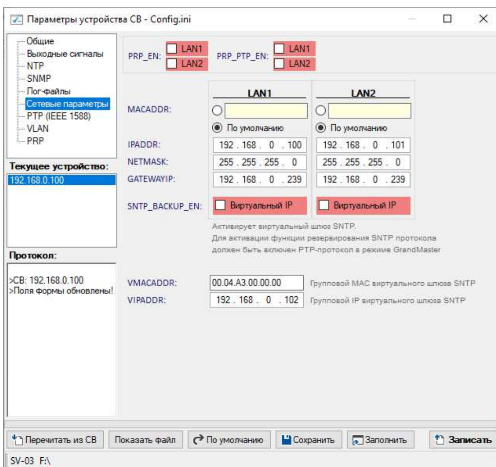
Рисунок 13 – Окно программы файла конфигурации (вкладка «Сетевые параметры»)
