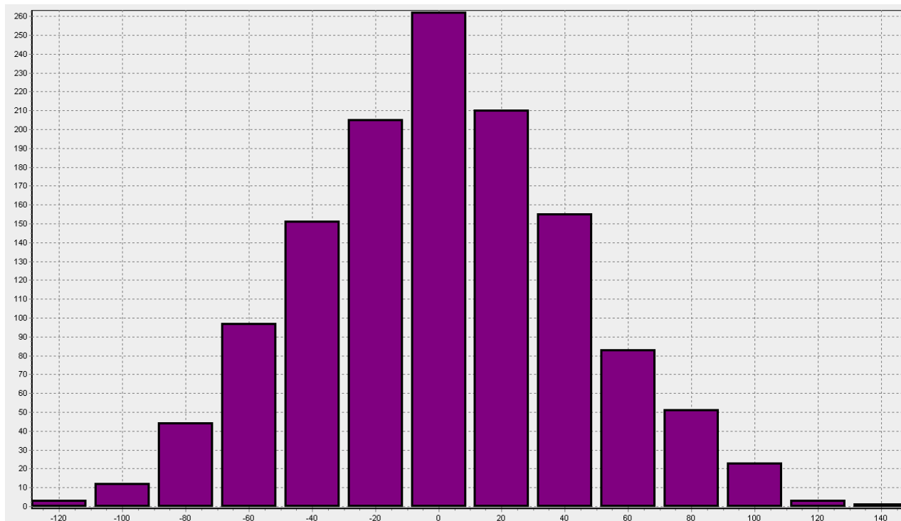
Рисунок 8 – Гистограмма распределения абсолютной ошибки синхронизации (нс) в режиме E2E GrandMaster – E2E Slave OC (между PTP устройствами включены «прозрачные» часы на базе RSG2288NC)
