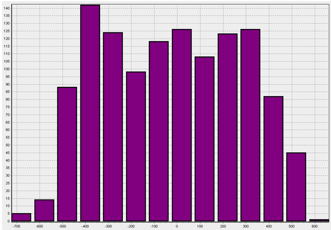
Рисунок 9 – Гистограмма распределения абсолютной ошибки синхронизации (нс) в режиме E2E GrandMaster – E2E Slave (между PTP устройствами включен pop - PTP свитч MOXA EDS-408A-MM-ST)
